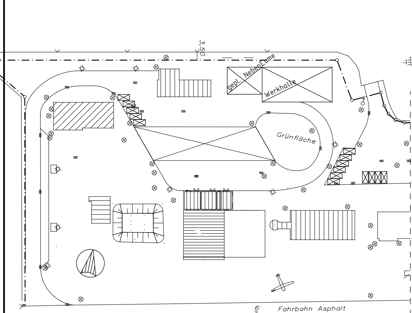
Lageplan : 1 - 1000
