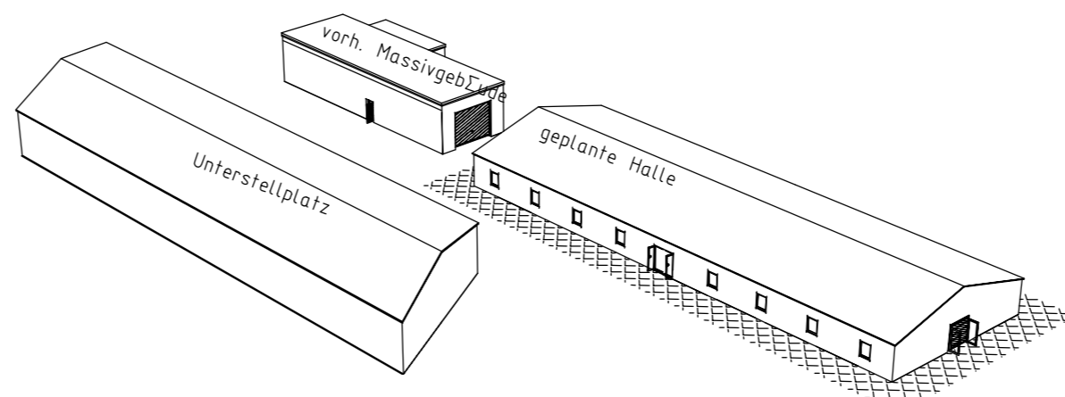
Ansicht Süd-Osten
